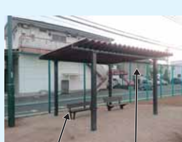
公園内休憩所改修 日よけ・椅子の設置
